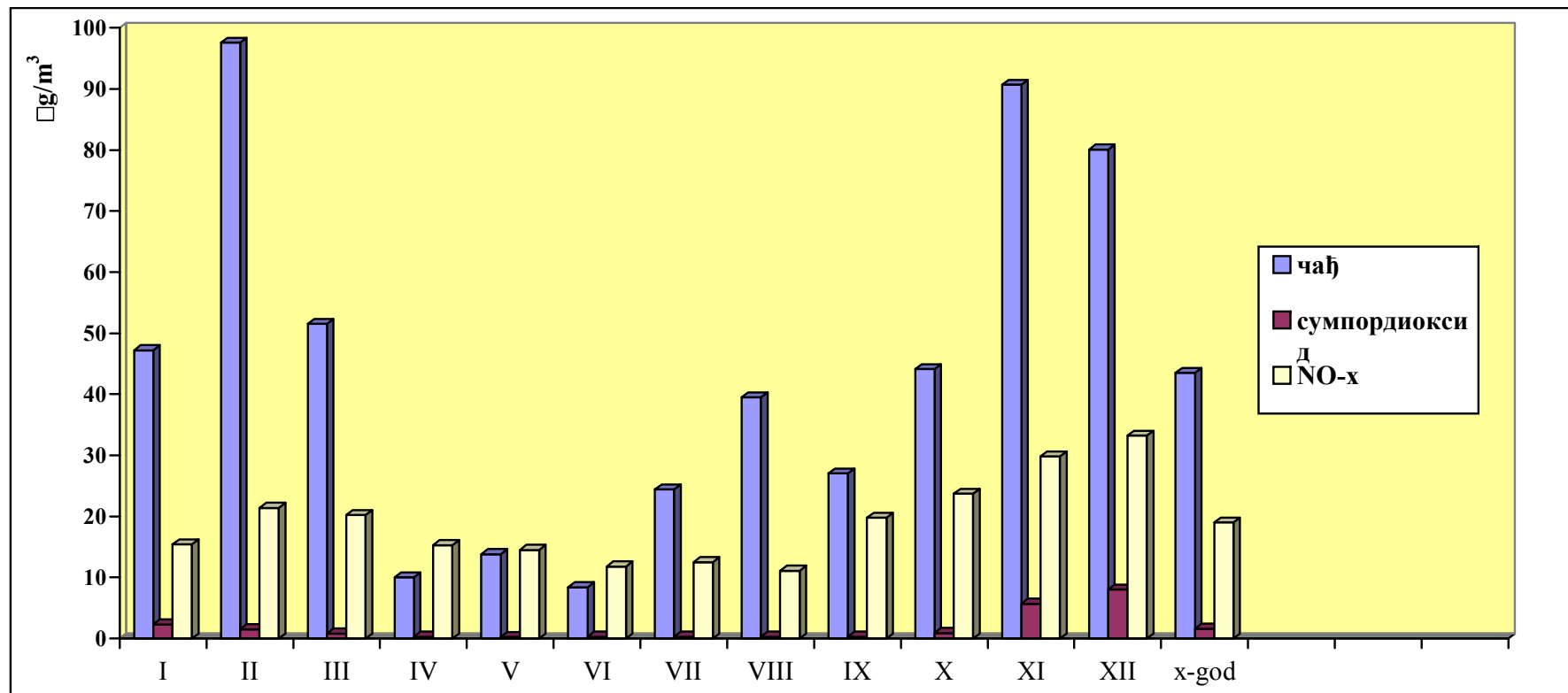
Слика бр.1. Хистограмски приказ кретања концентрације \text{SO}_2 , чађи и азотних оксида по месецима у 2012 години у Лесковцу на М.М.Бр.2-Летекс – Дунав центар
